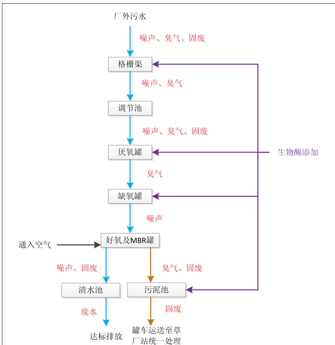
图 5-1 近期工艺流程及产污节点图
