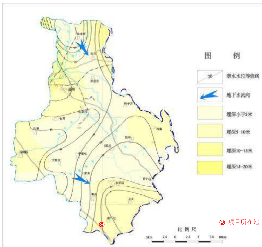
图 7-1 通州区潜水地下水水流场图
