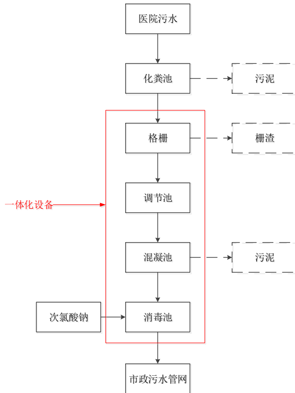
图 4-1 污水处理装置工艺流程图
