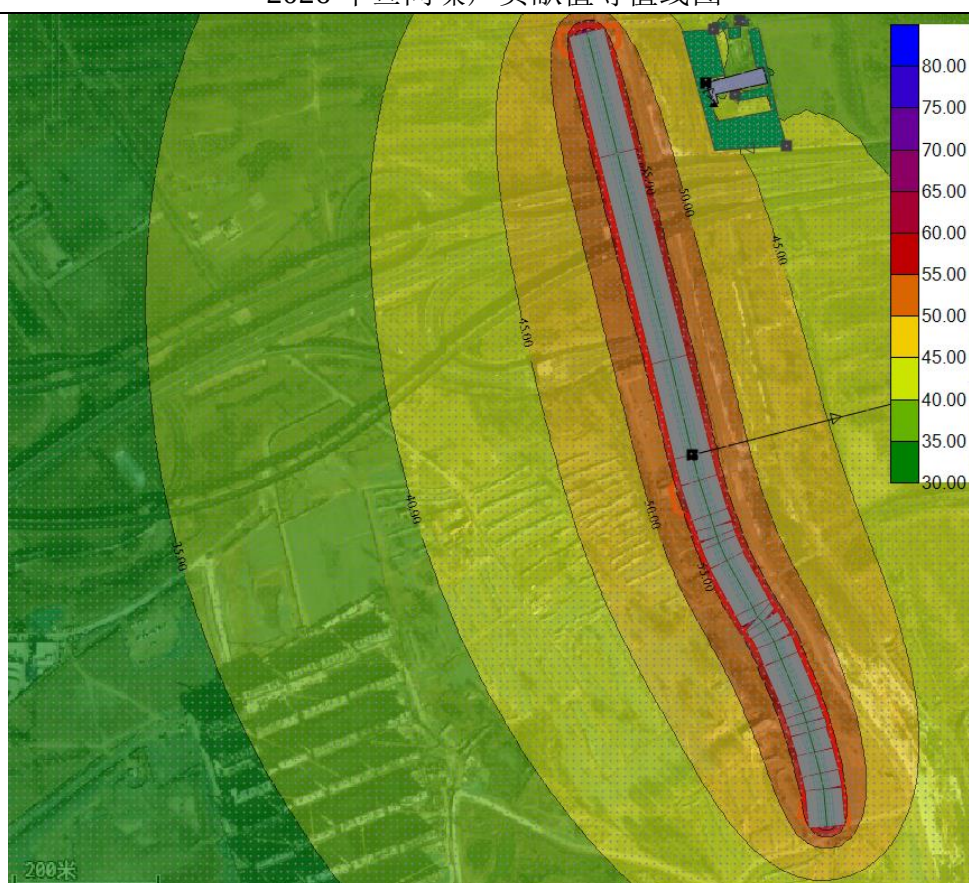
2026 年夜间噪声贡献值等值线图
