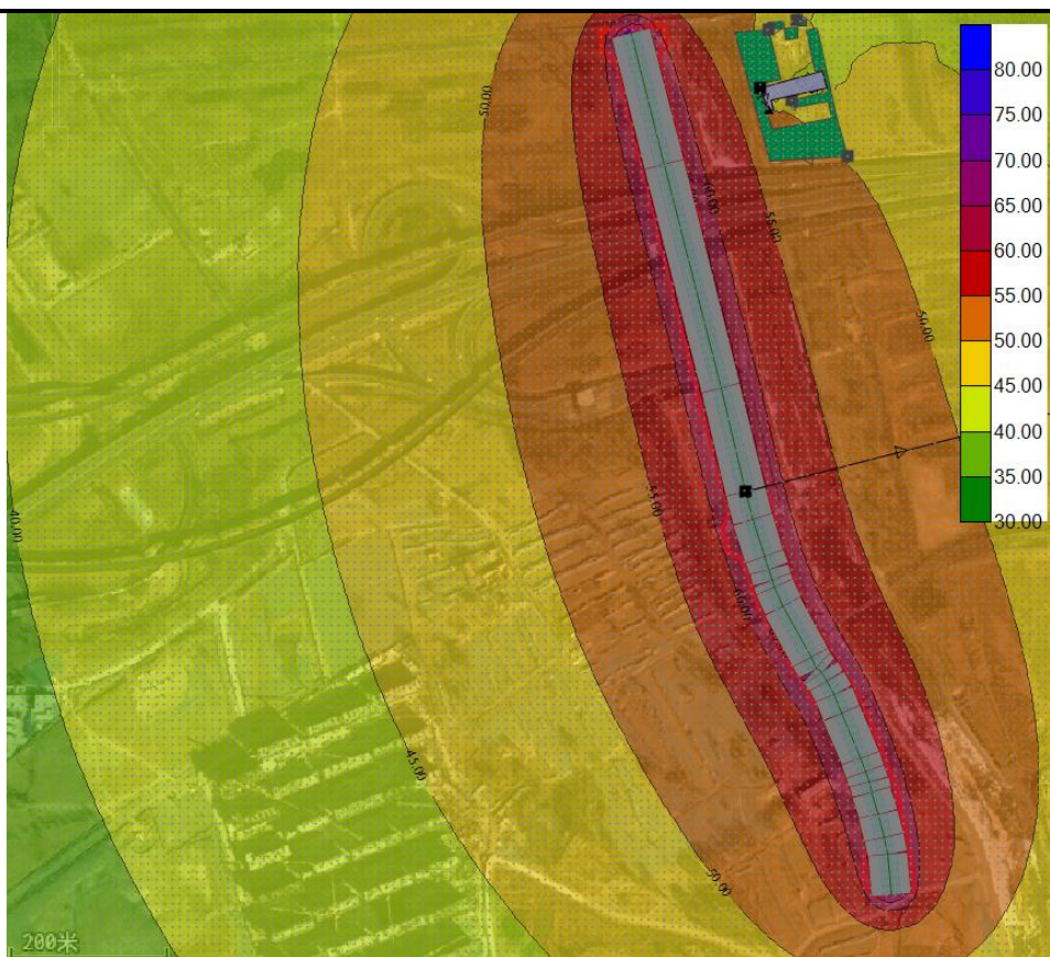
2032 年昼间噪声贡献值等值线图
