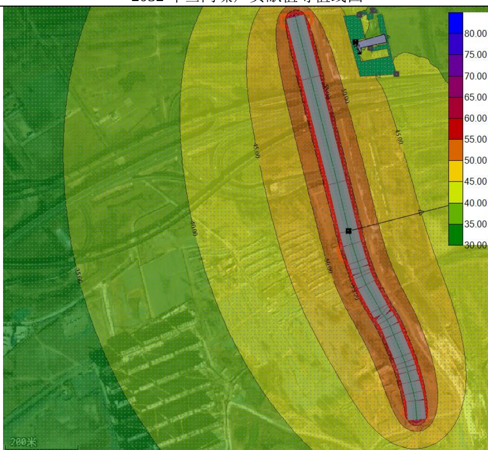
2032 年夜间噪声贡献值等值线图
