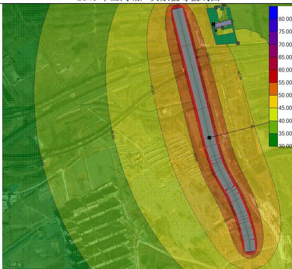
2040 年夜间噪声贡献值等值线图
