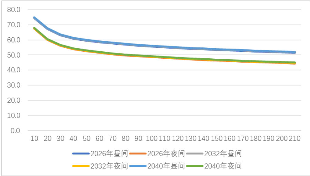
图 5-6 不同距离交通噪声衰减图
