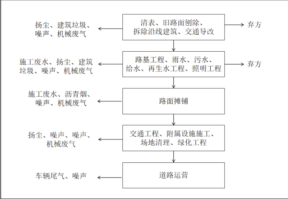
图 2-11 施工时序及产物节点示意图
