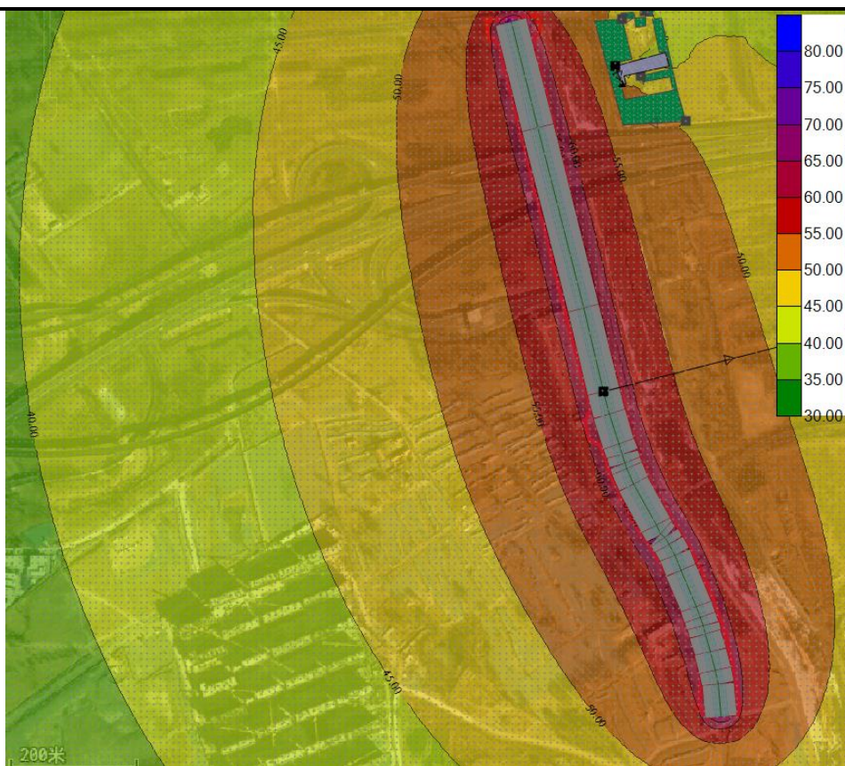
2026 年昼间噪声贡献值等值线图
