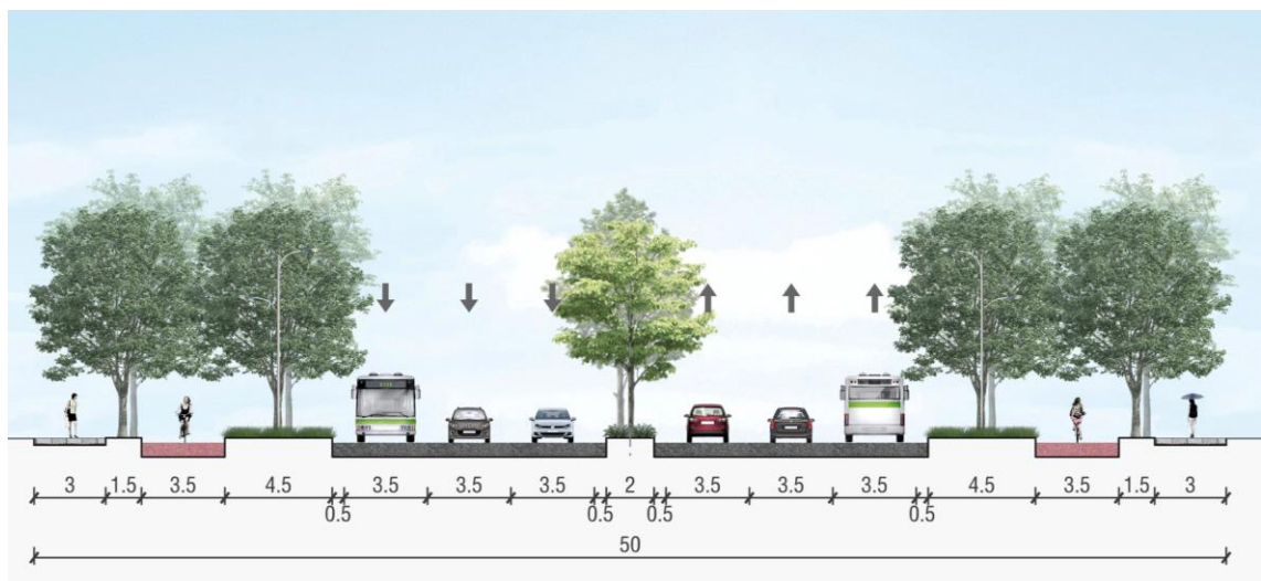
图 2-9 道路标准横断面图
