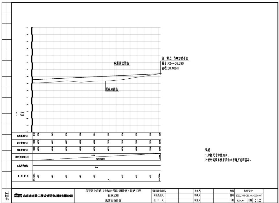
图2-8 道路标准纵断面图
