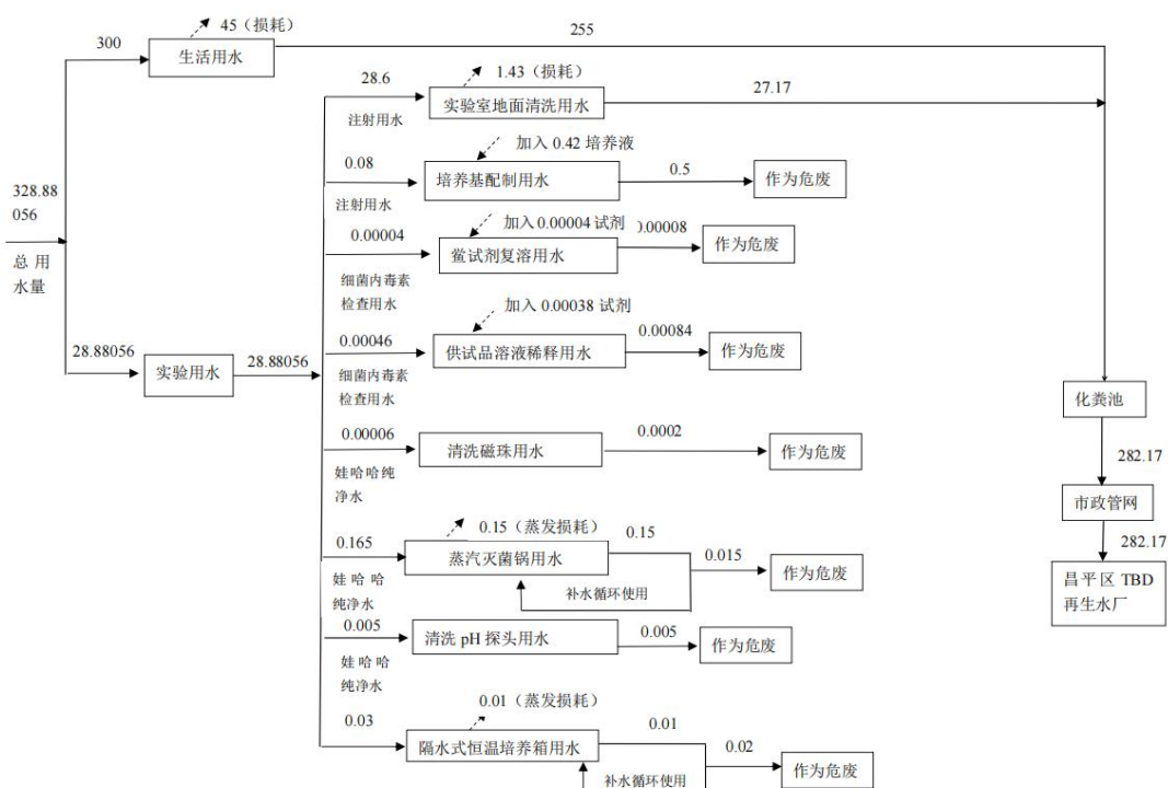
图 1 项目水平衡图 单位: m 3 /a
